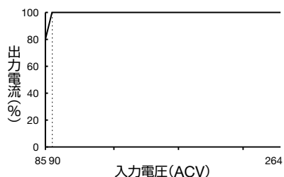
PS3V-015AF / -030AF形
