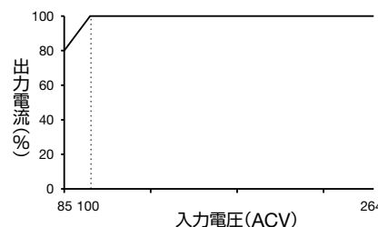
PS3V-100AF / -150AF形
