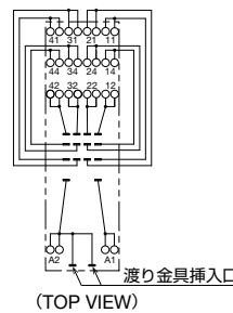
端子配列図
